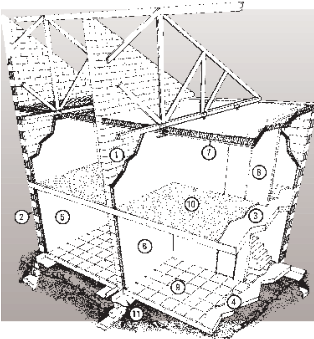
Mur simple en séparatif et dalle rez-de chaussée sur terre plein
