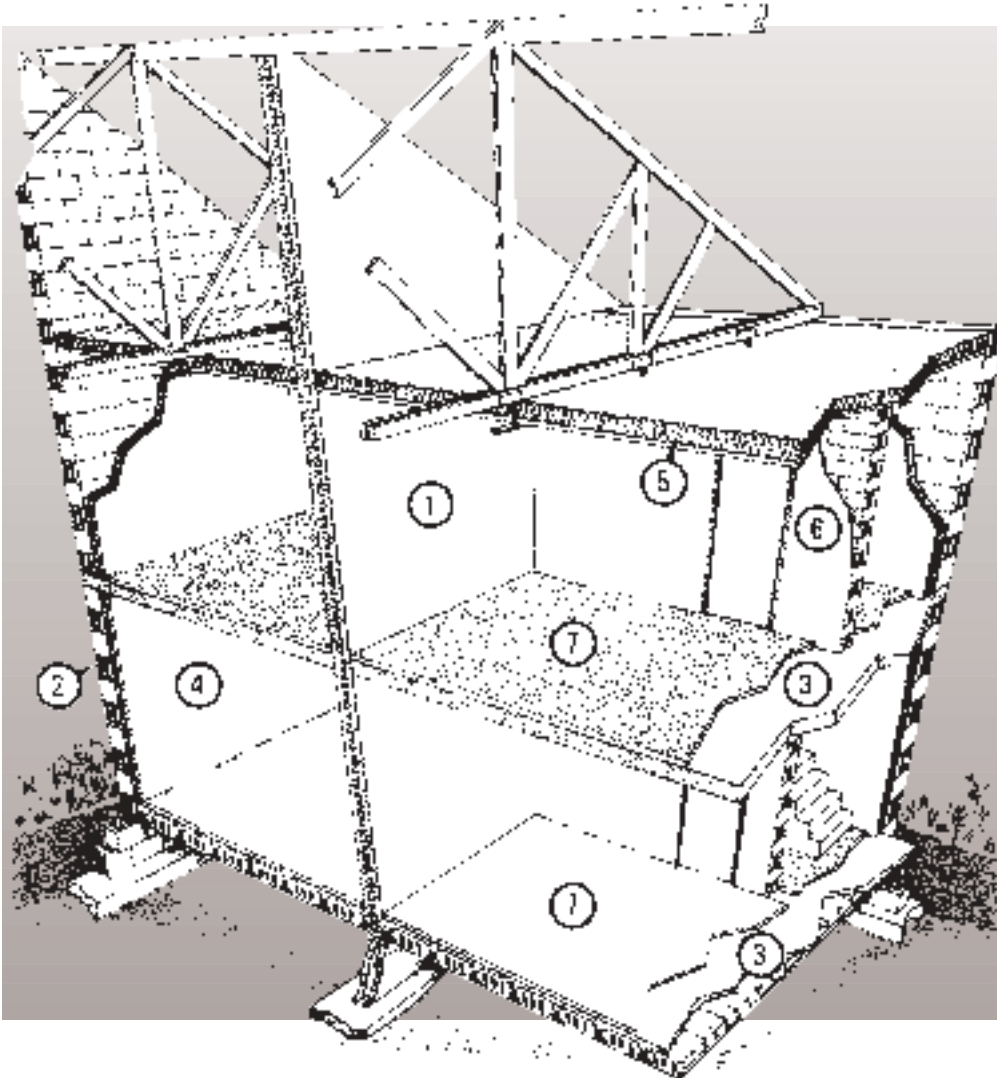
Mur double en séparatif
