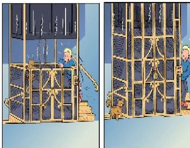
dispositif n°I-4 : clôture de gaine suffisante
